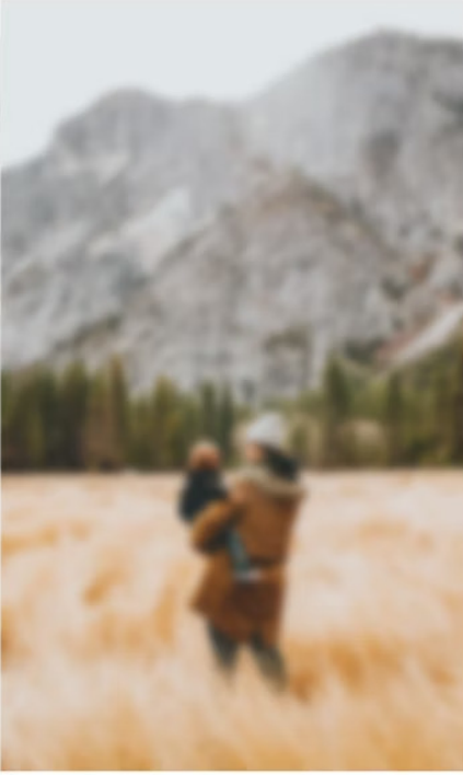
Astigmatismo
